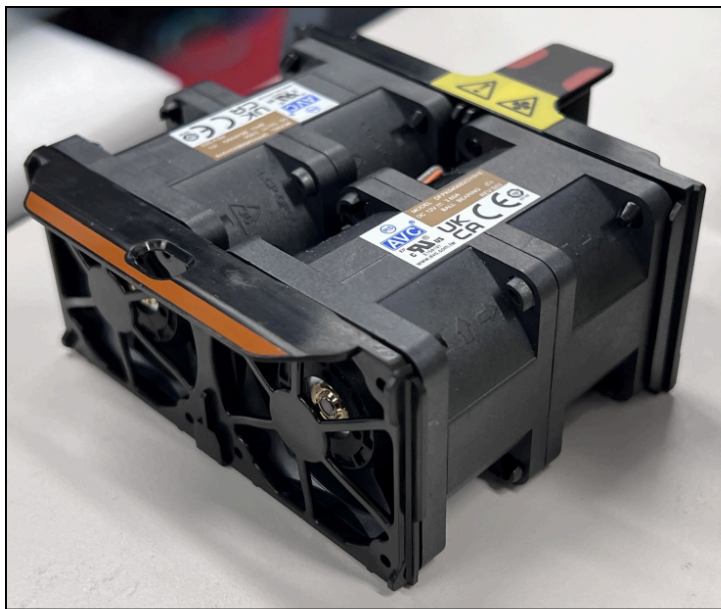
Figure 21. Fan module
